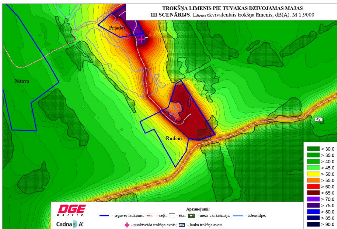
5.6.attēls. Trokšņu līmenis īstenojot trešo scenāriju.
