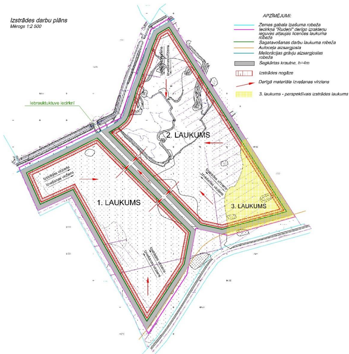
2.4.attēls. Izstrādes plāns pa ieguves posmiem iecirknī "Rudeņi".
