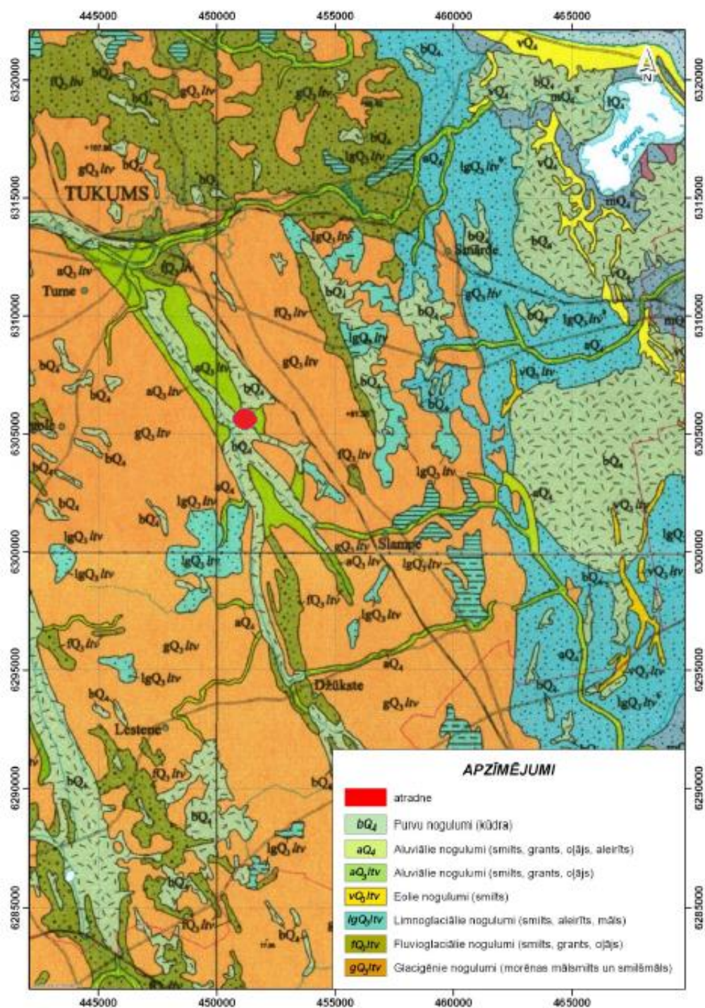
3.5.attēls. Kvartāra nogulumu karte.
