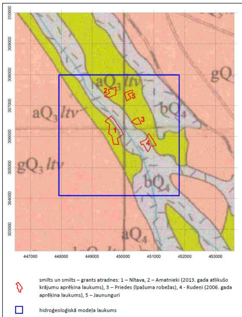
3.6.attēls. Atradņu atrašanās vietas kvartāra nogulumu kartē.
