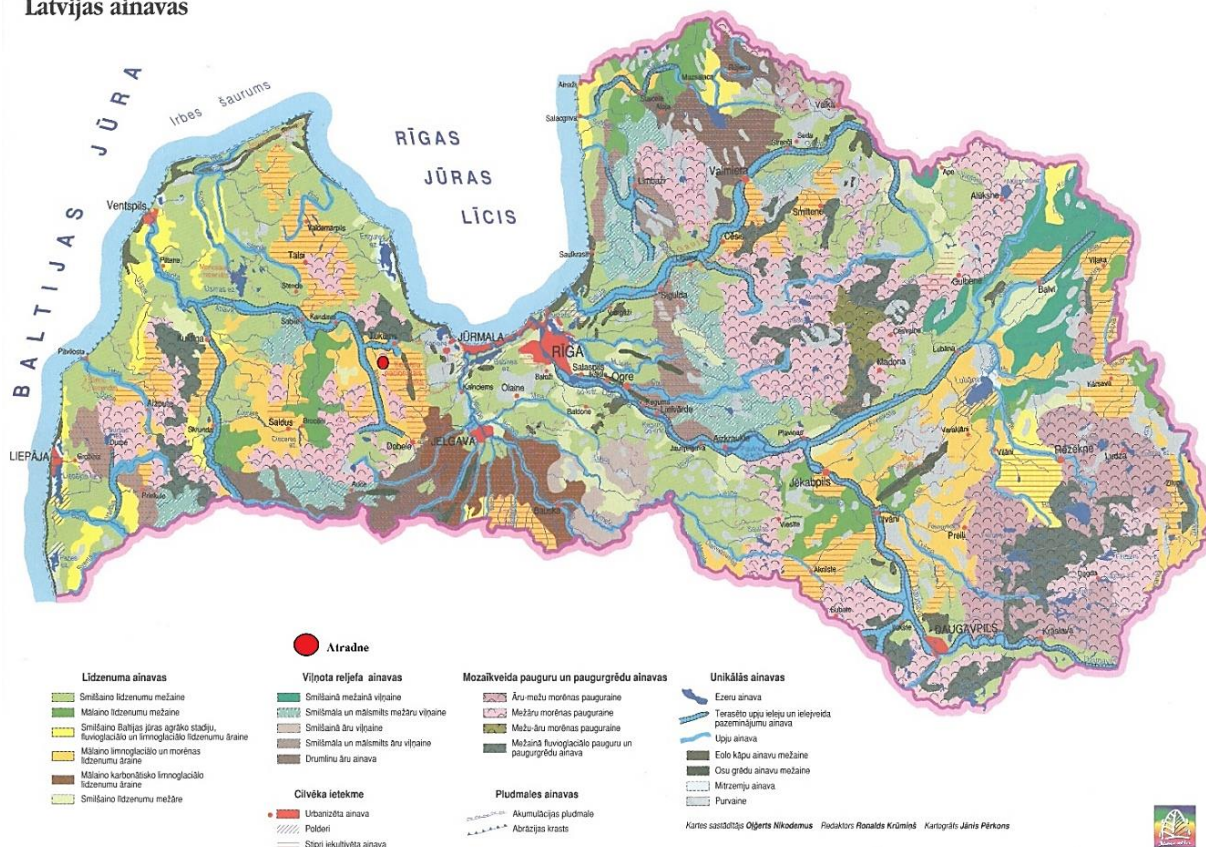
3.8.attēls. Latvijas ainavu karte 29 .
