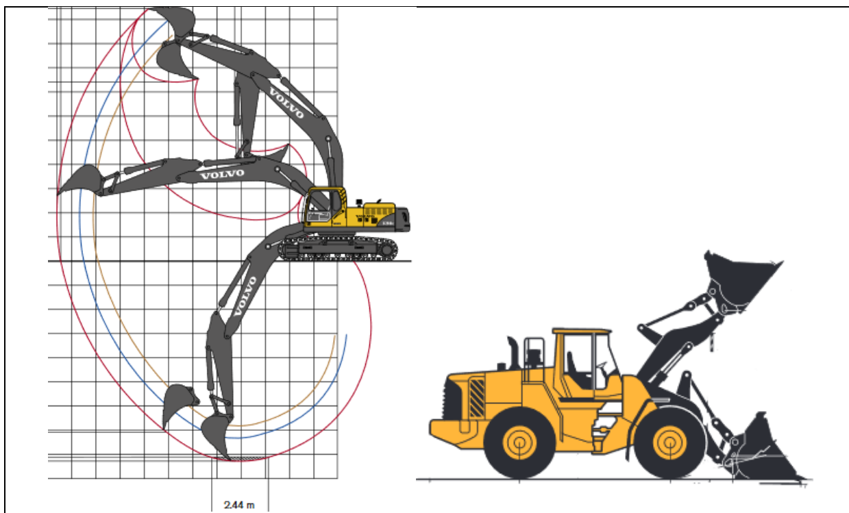
2.6.attēls. Ekskavators Volvo EC 290B (pa labi) 8 un frontālai iekrāvējs Volvo L180F (pa kreisi) 9 .
