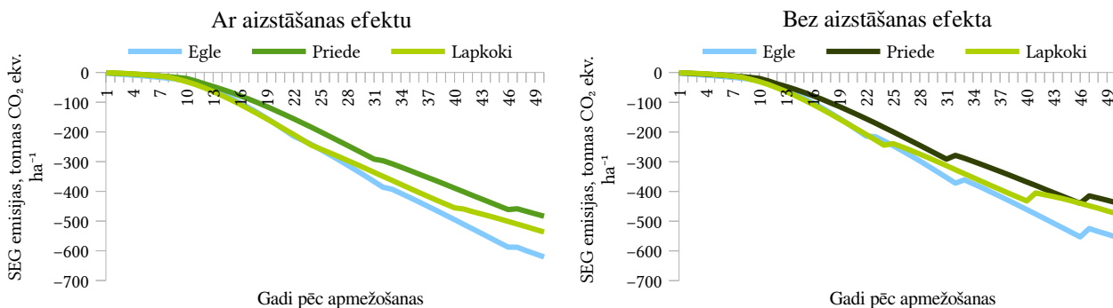
Att. 2. SEG emisijām apmežotajā platībā kumulatīvi, atkarībā no valdošās koku sugas.
