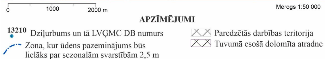
3.1.attēls Dziļurbumu izvietojuma shēma paredzētās darbības teritorijas apkārtnē
