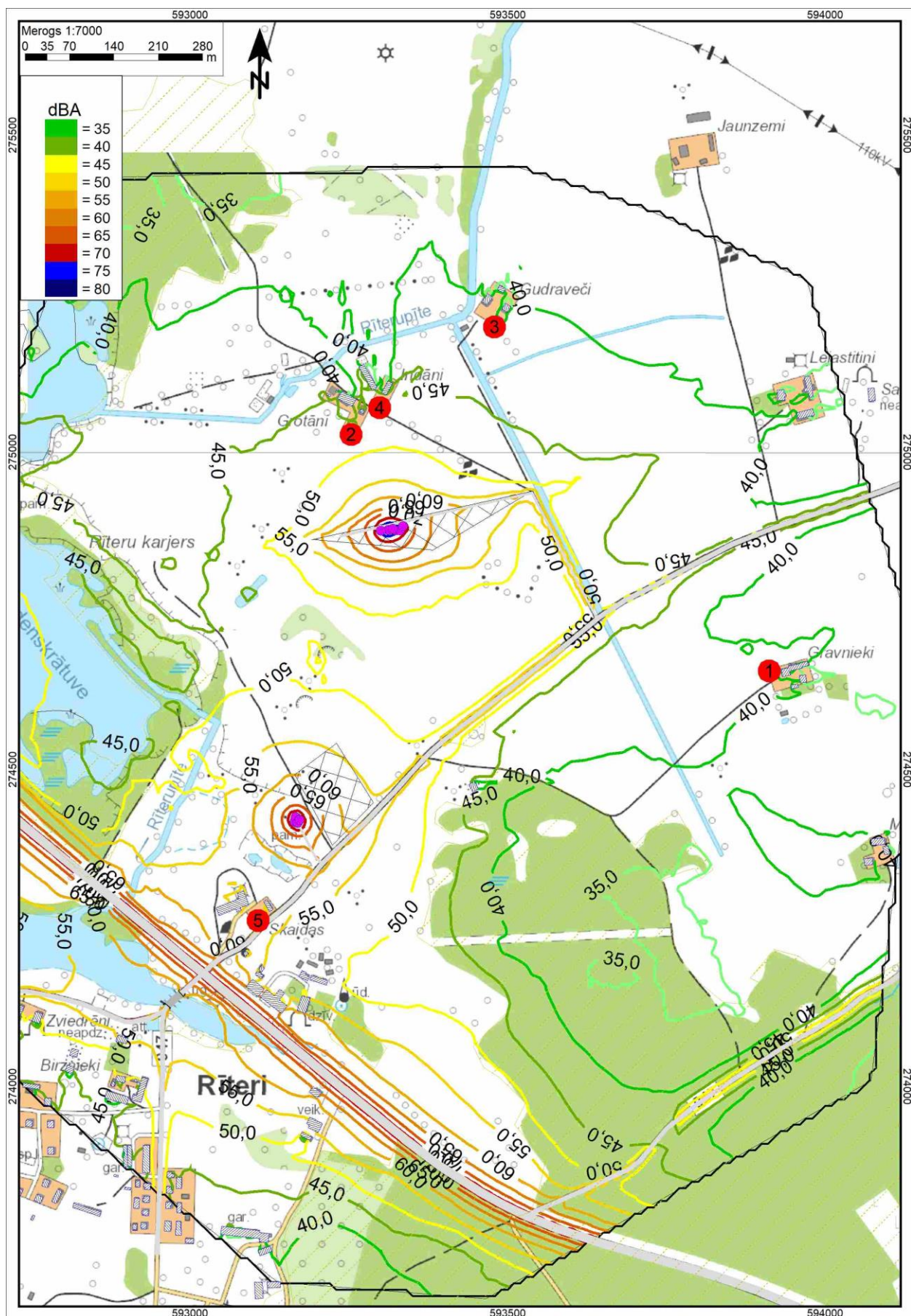
3.7. attēls. Trokšņa rādītāja L_{\text{diena}} aprēķinātās vērtības ar ieguvi 2. laukumā.
