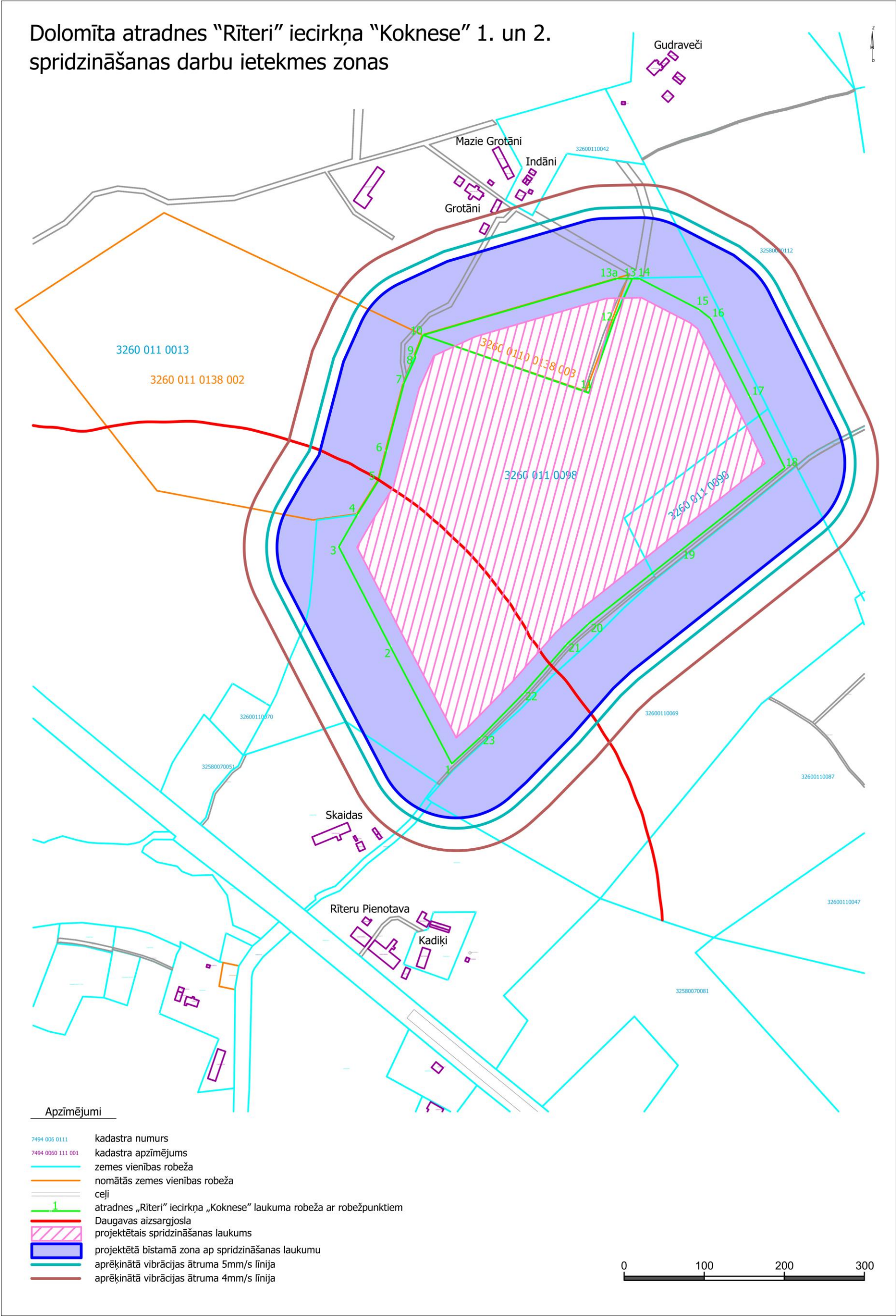
3.8. attēls. Dolomīta atradnes “Rīteri” iecirkņa “Koknese” 1. un 2. spridzināšanas darbu ietekmes zonas.
