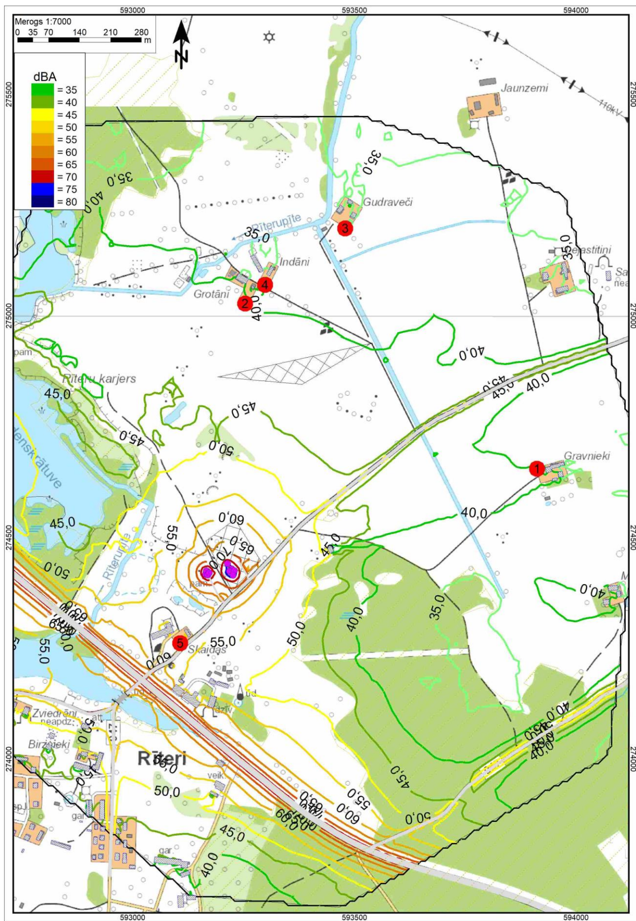
3.6. attēls. Troksņa rādītāja L_{\text{dienā}} aprēķinātās vērtības ar ieguvi 1. laukumā.
