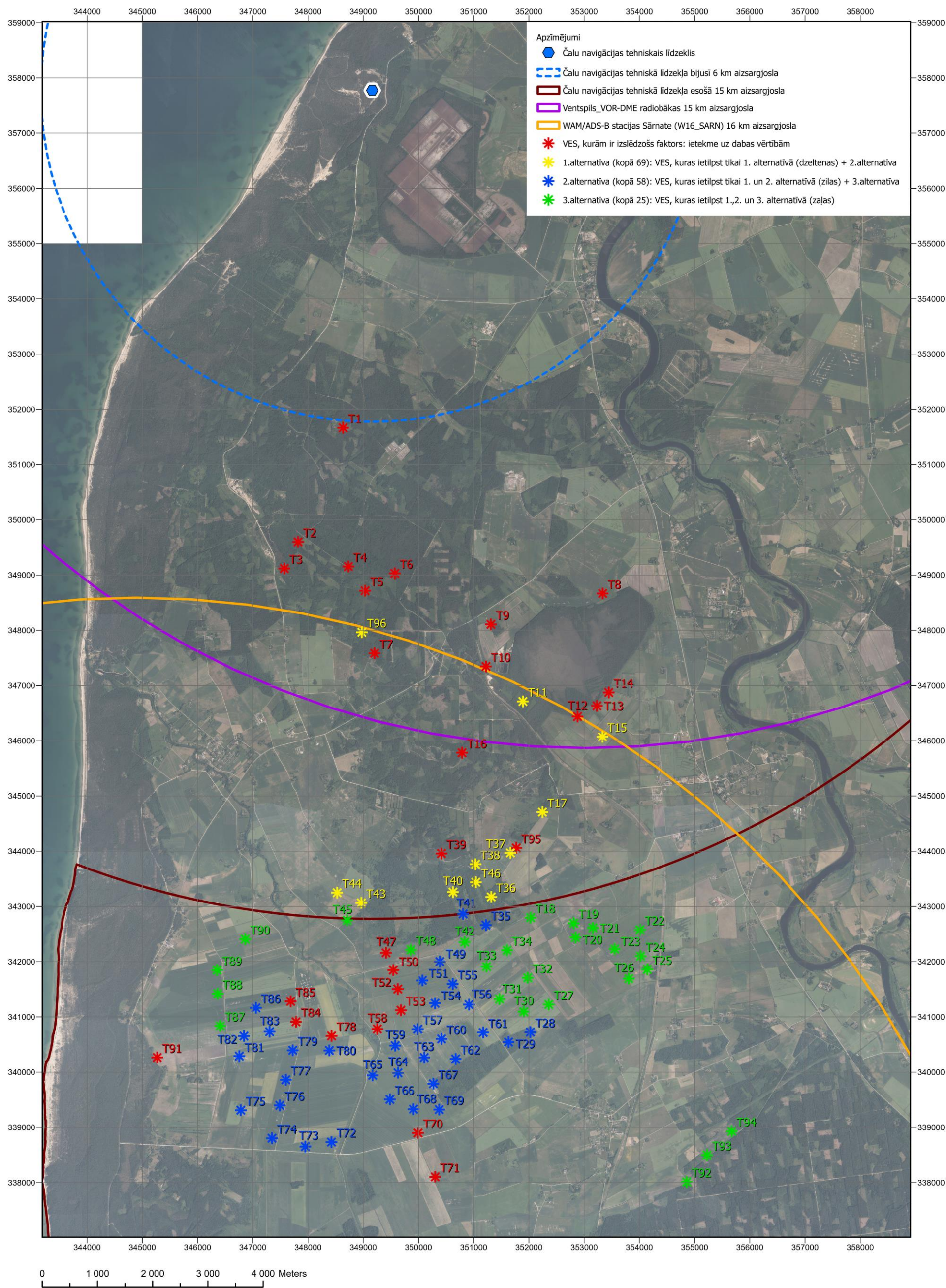
3.9. attēls. Valsts aizsardzības vajadzībām paredzētā Čalu navigācijas tehniskā līdzekļa un civilās aviācijas radiolokatoru aizsargjoslas (skaidrojumu par VES izvietojuma alternatīvām skat. tālāk 5. daļā).
