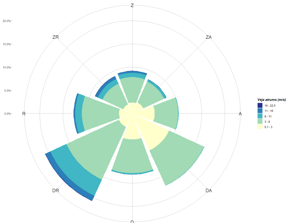
1.2. attēls. Vēja virziena atkārtošanās biežuma diagramma (vēja roze) ar vēja ātruma sadalījumu katram rumbam Ventspils novērojumu stacijā
